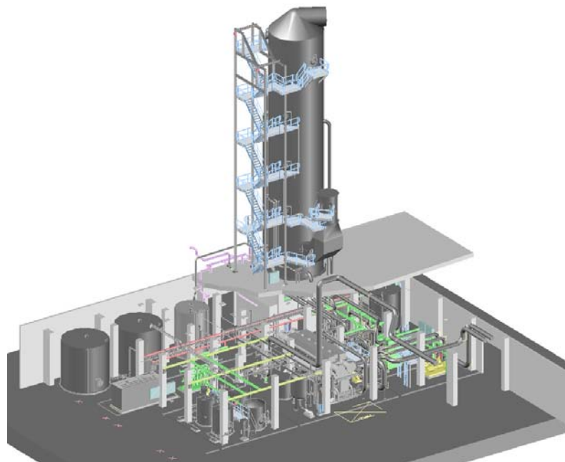
Helsingborg/Filborna plant Götaverken Miljö delivery
